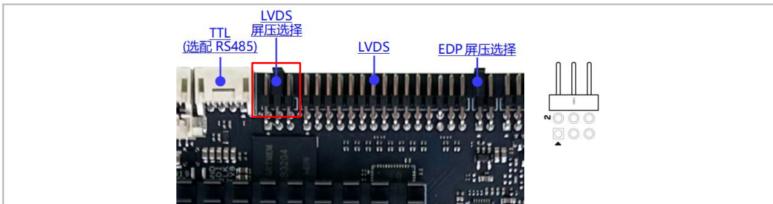
上图中用跳线帽来进行屏电源的选择
